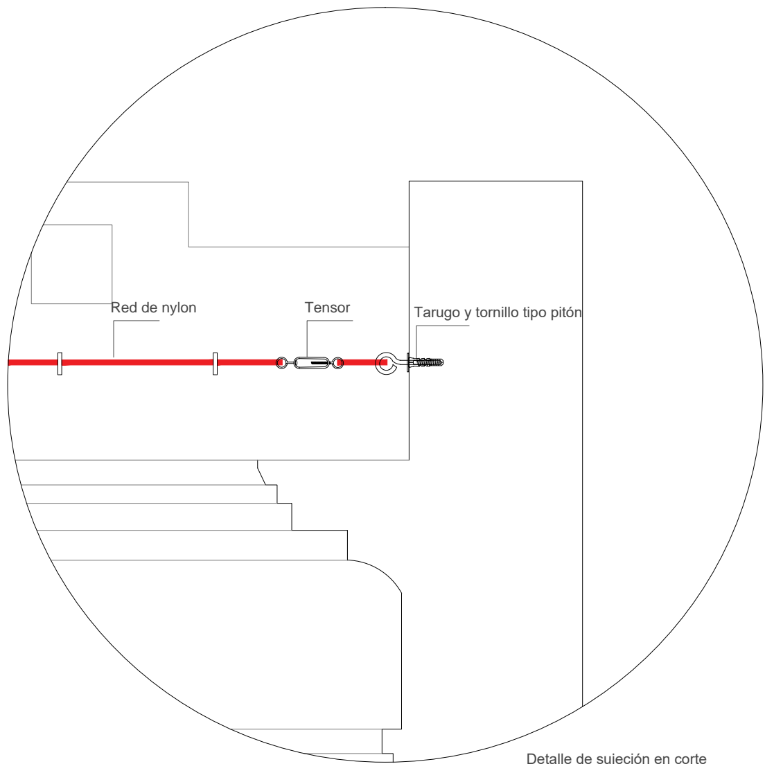
Detalle de sujeción en corte
