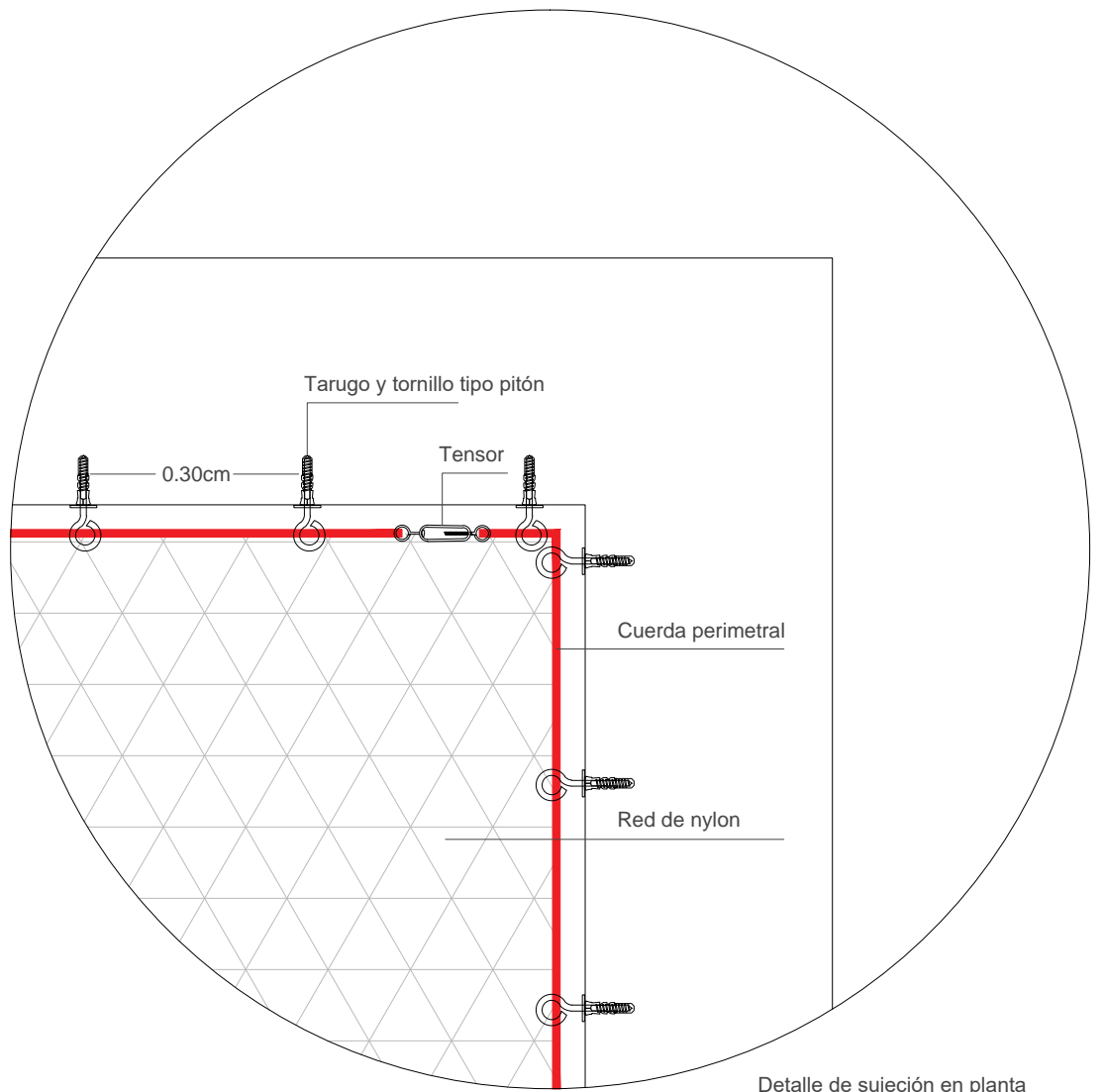
Detalle de sujeción en planta
